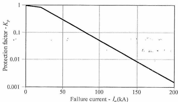
Hình A.2 - Hệ số bảo vệ ( K_p ) là hàm của dòng gây hư hỏng ( I_a )
