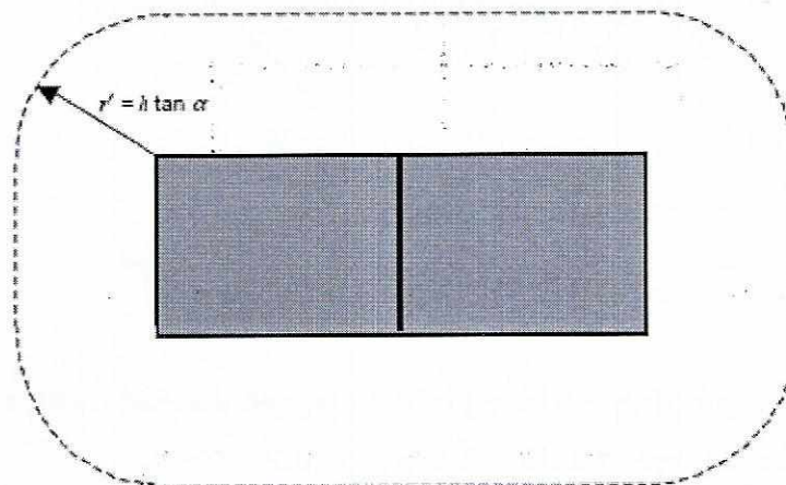
Hình B.5 - Vùng được bảo vệ bởi các dây dẫn dạng lưới không tách biệt, xác định theo phương pháp mặt lưới và phương pháp quả cầu lăn
